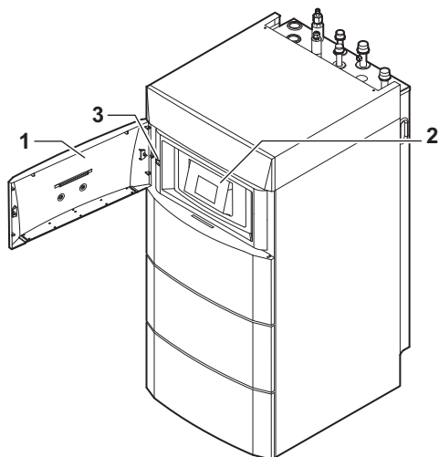
Obr.3 Hlavní součásti
